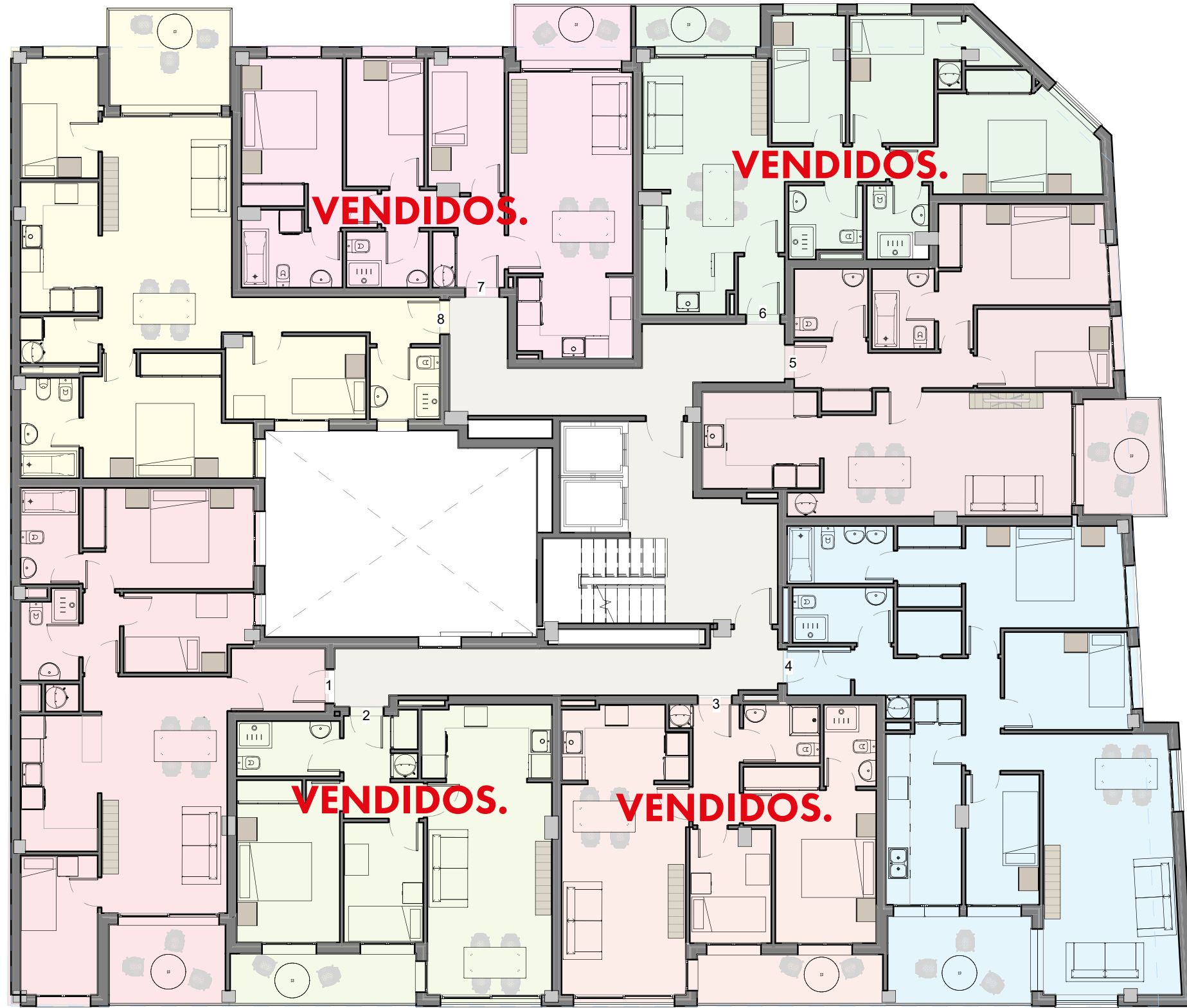
01 Planta primera-DAU A3 1_125 Copia 1 1 : 125
